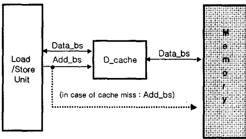
그림 2. 메모리 시스템 구조
