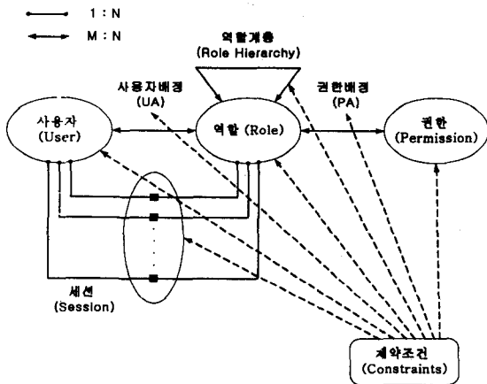
그림 1. RBAC 모델
