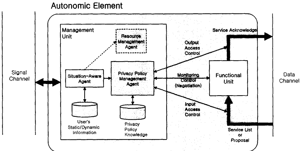
그림 1. 개인정보보호를 위한 오토노믹 엘리먼트 아키텍처 구성도
