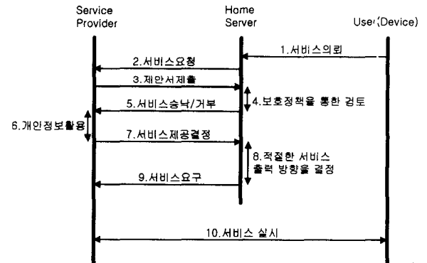
그림 2. 서비스 제공을 위한 각 개체들의 상호작용
