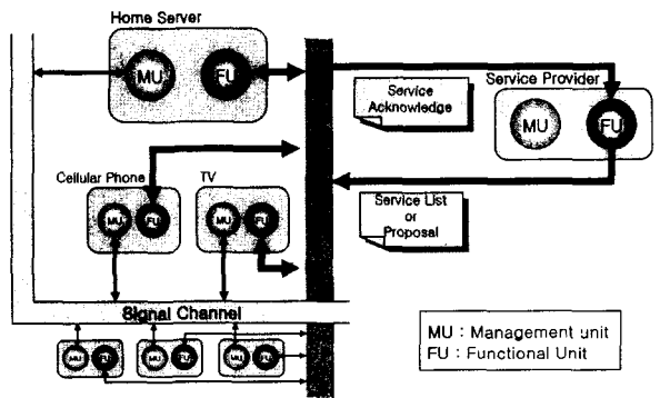
그림 3. 다른 오토노믹 엘리먼트들 간의 상호작용
