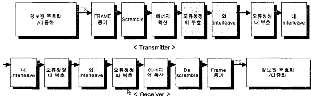
그림 2 FPU시스템의 송·수신 구조
