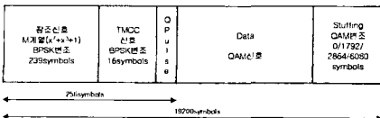
그림 4. 파형등화용 기준신호의 Format
