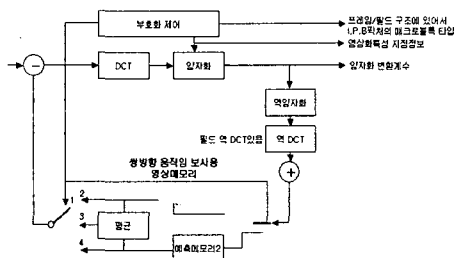
그림 1. MPEG-2의 부호기
