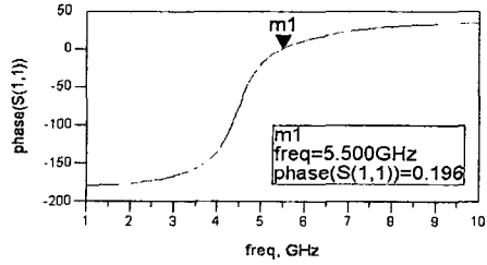
(b) S11 위상 변화
