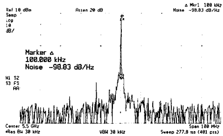
(c) 위상 잡음 그림 9. 발진기 출력 특성
