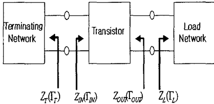
그림 4. 2단자망 발진기 블록도
