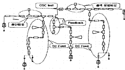
그림 6. 발진 가능성 테스트를 위한 회로
