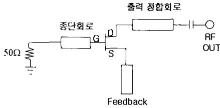
그림 5. 발진기 구조
