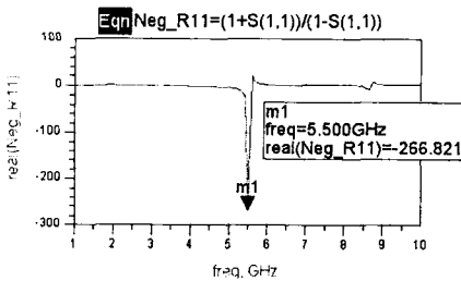
그림 4. 부성저항 특성
