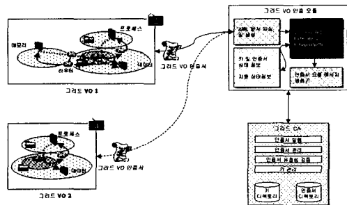
그림 5. 그리드 VO 인증 시스템의 전체 구조
