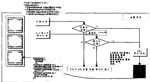
그림 6. 그리드 VO 인증 모듈의 전체적인 구조
