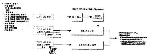
그림 7. XML 서명 문서 생성
