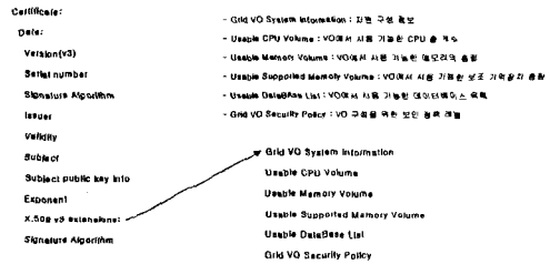
그림 11. 그리드 VO 인증서의 필드 형식
