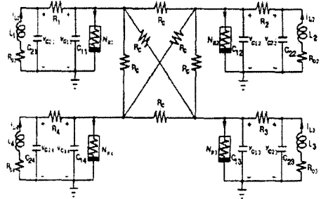
그림 3. Chua's 회로를 이용하여 구성한 Small World 네트워크
