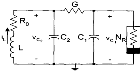
그림 2. Chua's 회로
