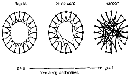
그림 1. 정규 네트워크, small world, 랜덤 네트워크 비교
