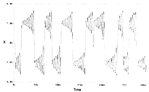
(b) v_{c2} 단의 시계열 데이터
