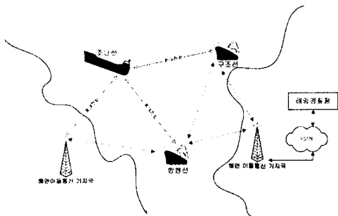
그림3-1. 육상이동통신시스템의 해상 확장
