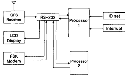
그림-10 데이터취득, ID set 및 전송부 블록도
