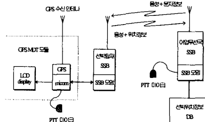
그림-3 SSB모뎀형 GPS-MDT의 운용
