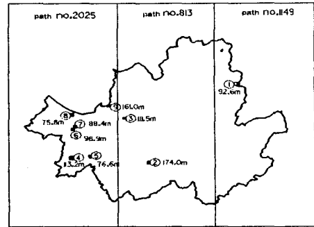
그림 6. 기준점의 위치 및 표고
