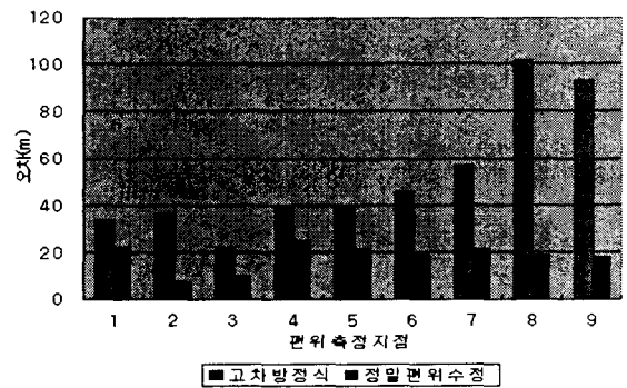
그림 7. 기준점과 영상간의 편위 오차
