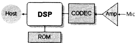
그림 2. VR-33R 블록 다이어그램
