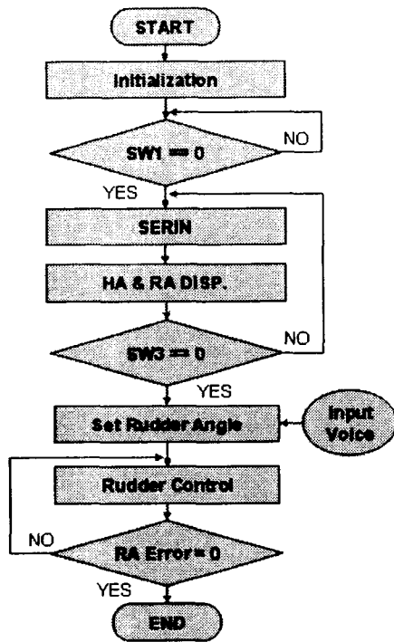
그림 5. 조타제어 프로그래밍 흐름도
