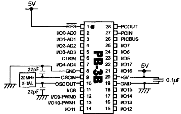
그림 3. PB-3B 연결도
