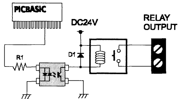
그림 4. 릴레이 제어 회로
