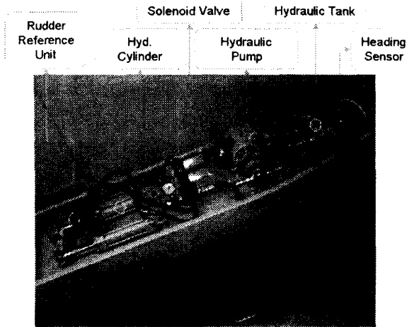
그림 7. 모형선박의 조타시스템 구성
