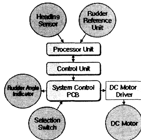
그림 6. 자동조타 및 시스템 제어 장치 구성
