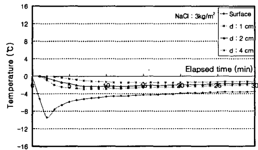
그림 2 NaCl 분말 살포시 콘크리트 단면의 온도변화
