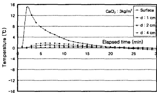
그림 1 CaCl 2 분말 살포시 콘크리트 단면의 온도변화
