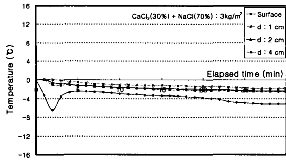
그림 3 혼합 분말 살포시 콘크리트 단면의 온도변화
