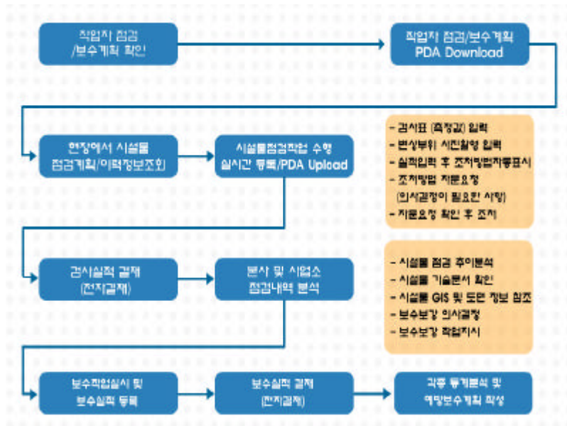
그림 1. 도시철도 설비시설물 유지보수업무 표준 절차
