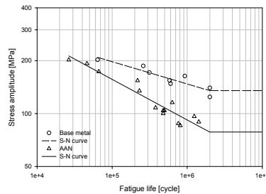
Fig. 5 BM and AAN
