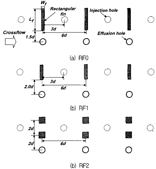
Fig. 2 Fin configurations
