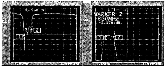
그림 7. BPF 2 반사손실과 삽입 손실 특성 (Marker 1 : 500 MHz, Marker 2 : 850 MHz).
