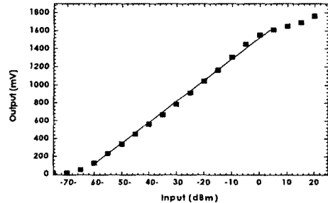
그림 9. 영상검출기의 입출력 특성 ( y = 23.4x + 1519 ).
