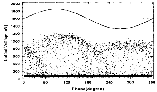
(c) BPF 3을 사용한 경우의 PRPD Pattern.
