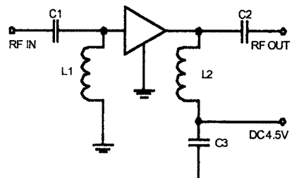
그림 2. 광대역 저잡음 증폭기 회로도.
