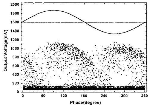
그림 13. 3 pC PD에 대한 극초단파 신호처리장치의 PRPD Pattern (BPF 1을 적용, 1200주기).
