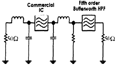
그림 3. BPF 1, 2 구성도.
