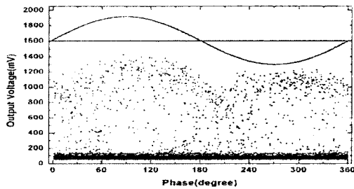
(a) BPF 1을 사용한 경우의 PRPD Pattern.
