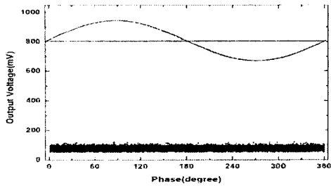
(a) 극초단파 신호처리장치의 내부 잡음.
