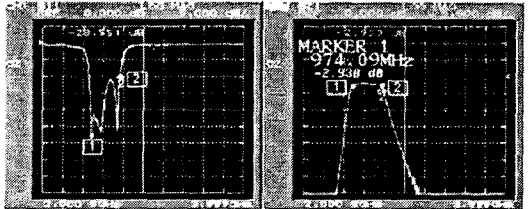
그림 8. BPF 3의 반사손실과 삽입 손실 특성 (Marker 1 : 974 MHz, Marker 2 : 1600 MHz).
