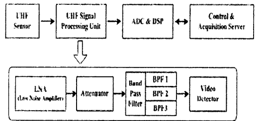
그림 1. GIS용 PD 감시시스템의 구성도와 UHF신호처리장치의 상세 블록도.
