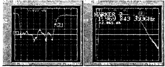
그림 6. BPF 1의 반사손실과 삽입 손실 특성 (Marker 1 : 300 MHz, Marker 2 : 1970 MHz).
