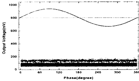
(b) 센서를 연결하고 PD 신호가 없을 경우의 주변잡음.
