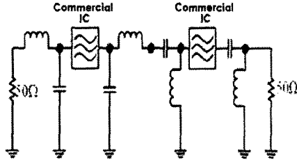
그림 4. BPF 3의 구성도.
