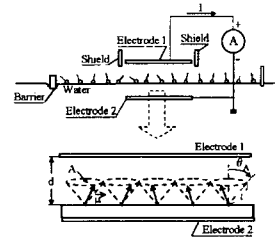
그림 1 변위전류 측정장치
