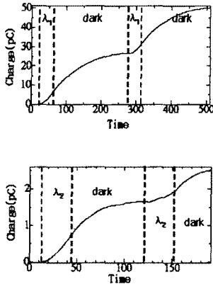
그림 7. AZ-G4의 전하량( \lambda_1=365\text{nm}, \lambda_2=450\text{nm} ) Fig. 7. Change of AZ-G4( \lambda_1=365\text{nm}, \lambda_2=450\text{nm} )
