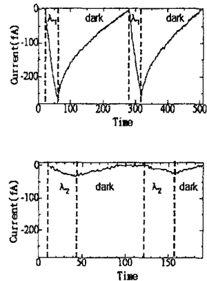
그림 6. AZ-G4의 광조사( \lambda_1=365\text{nm}, \lambda_2=450\text{nm} ) Fig. 6. Photoirradiation of AZ-G4( \lambda_1=365\text{nm}, \lambda_2=450\text{nm} )
