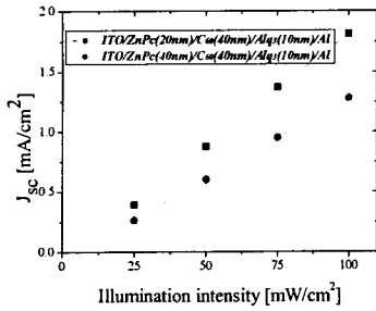
그림 7. ITO/ZnPc/C 60 /Alq 3 /Al 소자의 단락전류.
