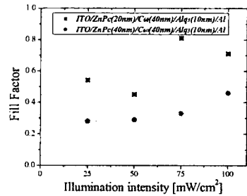
그림 6. ITO/ZnPc/C 60 /Alq 3 /Al 소자의 Fill factor.
