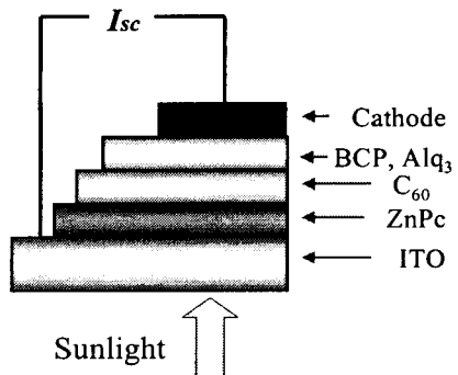
그림 2. 유기 광기전 소자의 구조.
