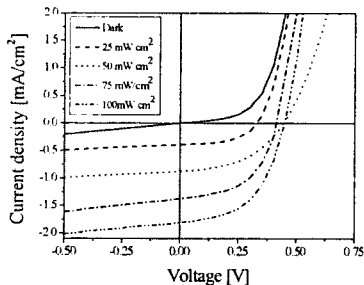
그림 4. ITO/ZnPc/C 60 /Alq 3 /Al 소자의 전압-전류 특성.
