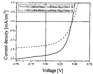
그림 5. ZnPc 두께 변화에 따른 PV 특성.
