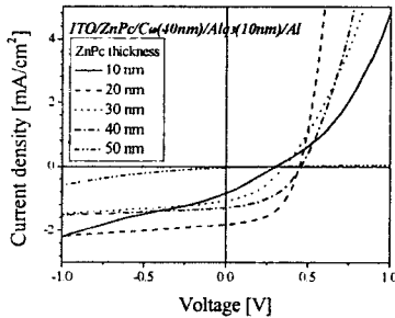
그림 3. ZnPc 두께 변화에 따른 PV 특성.
