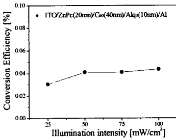
그림 8. ITO/ZnPc/C 60 /Alq 3 /Al 소자의 변환 효율.
