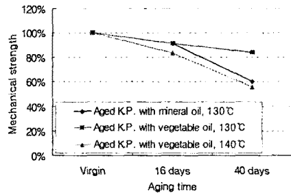
그림 2. 열화 절연유 종류 및 열화시간에 따른 절연지의 인장강도 특성 비교
