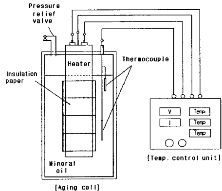
그림 1. 가속열화 모의 시험장치 구성
