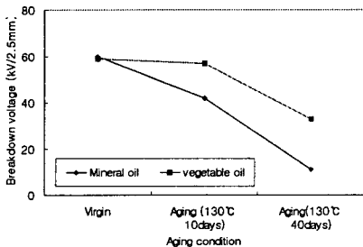
그림 5. 절연유의 열화에 따른 절연내력 변화
