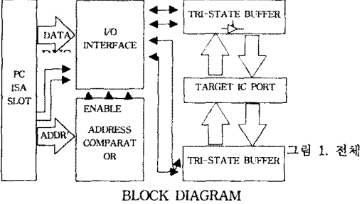
그림 1. 전체 BLOCK DIAGRAM
