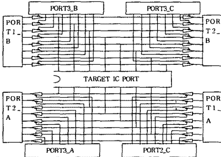
그림 3. TRI-STATE BUFFER BOARD 회로도
