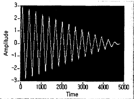
그림 4. 탈자 파형
