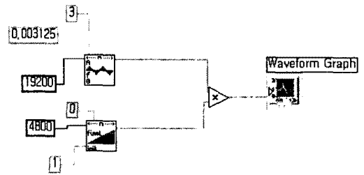
그림 5. 탈자 프로그래밍 블록도
