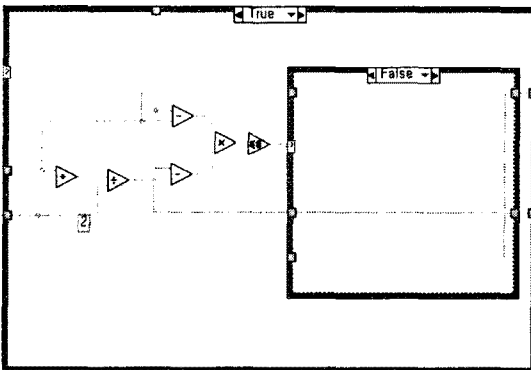
그림 4. 2분활법 알고리즘 블록도
