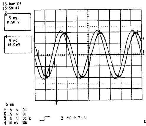
그림4(d) 인버터 출력 전압 및 전류(50kW)
