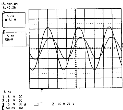
그림4(c) 인버터 출력 전압 및 전류(15kW)
