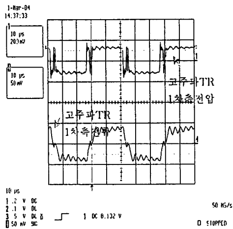
그림2(b) 고주파변압기 입력 전압 및 전류
