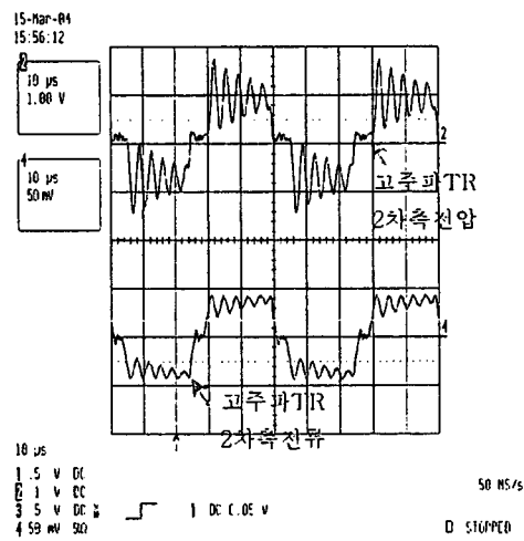
그림2(d) 고주파변압기 출력 전압 및 전류
