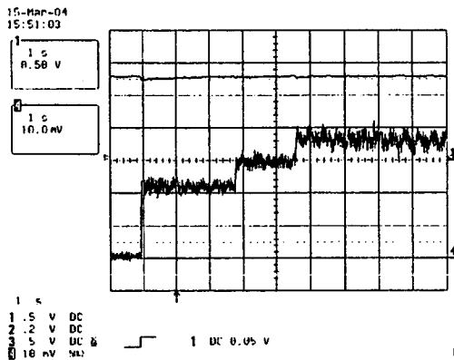
그림3. 부하변경시 컨버터 출력전압과 전류
