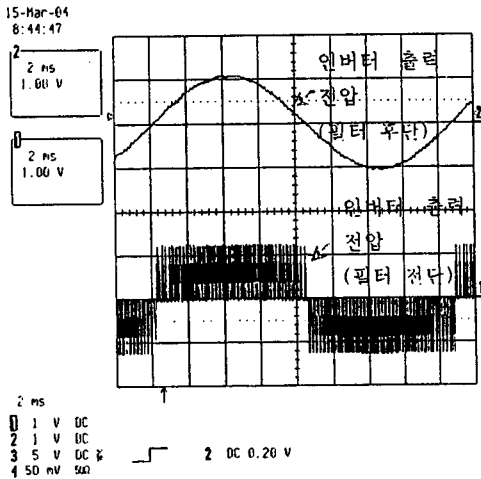
그림4(a) 인버터 출력필터 전/후단 전압 파형
