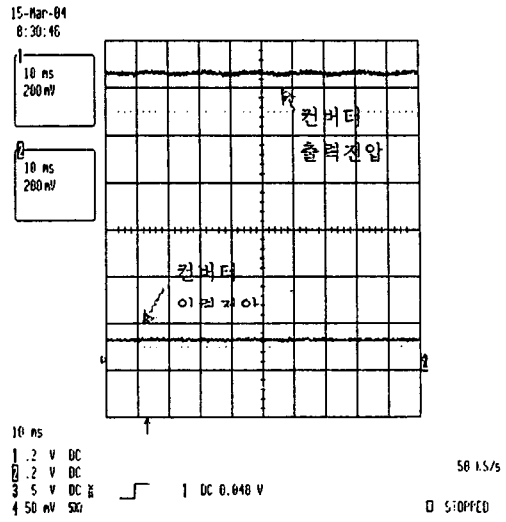
그림2(f) 컨버터 입력 및 출력 전압
