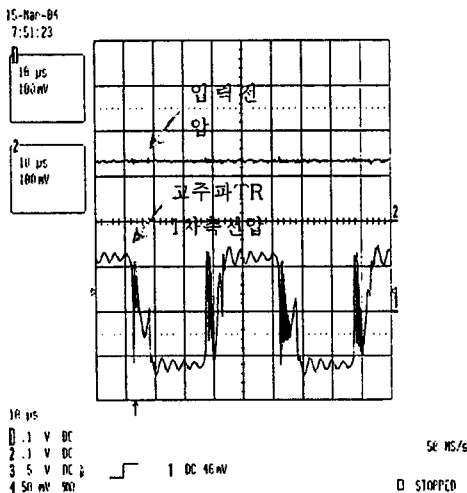
그림2(a) 컨버터 및 고주파변압기 입력전압
