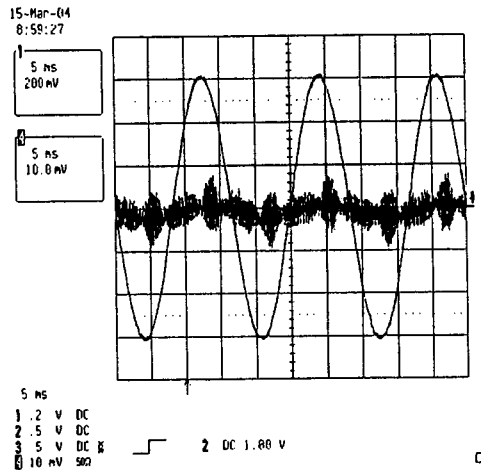
그림4(b) 인버터 출력전압 및 필터 유입전류
