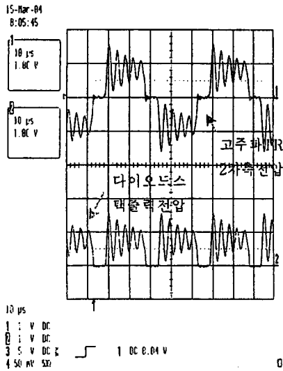
그림2(e) 고주파변압기 및 다이오드스택 출력
