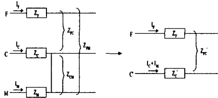
그림 7. 전차선로 임피던스의 등가화
