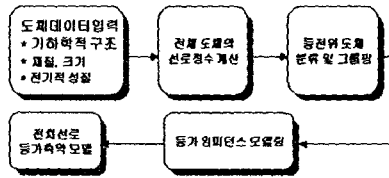
그림 3. 선로정수 계산 과정
