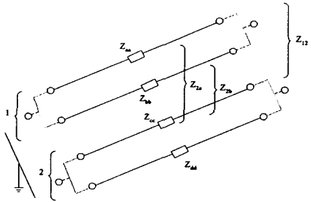
그림 6. 도체 그룹 사이의 상호 임피던스
