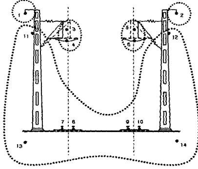
그림 1. 전차선로의 기하학적 구조
