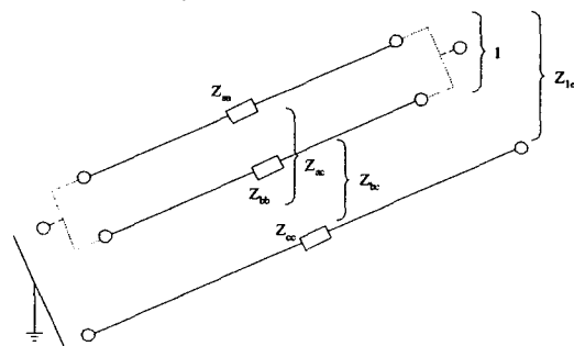
그림 5. 도체 그룹과 도체 사이의 상호 임피던스
