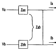
그림 4. 도체 그룹의 자기 임피던스
