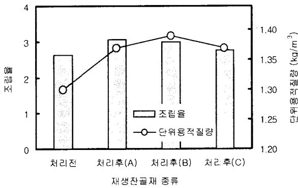
(a) 조립율 및 단위용적질량
