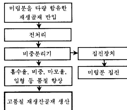
그림 1. 재생잔골재 생산 시스템의 개요
