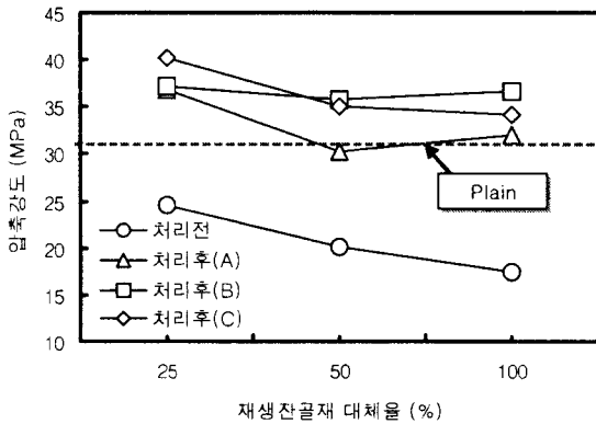
그림 5. 재생잔골재 종류에 따른 압축강도 성상 (재령 28일)
