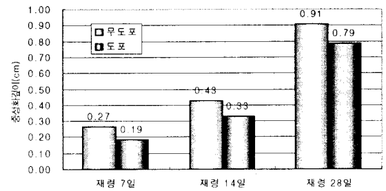
그림 7. 촉진중성화 깊이
