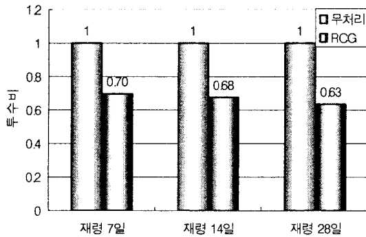
그림 1. 투수시험 결과
