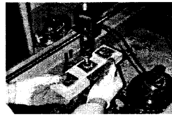
사진 1. 탈락강도 측정 상황
