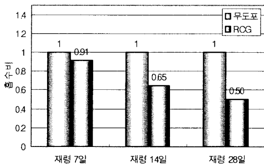
그림 2. 흡수시험 결과
