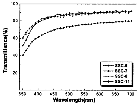
그림 3. Spectrophotometer를 이용한 4종류의 ITO 필름의 투과율.
