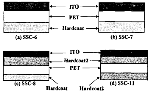
그림 1. 사용한 4종류의 ITO 필름의 픽셀 구조. Fig. 1. The structure of four other ITO film fixels.
