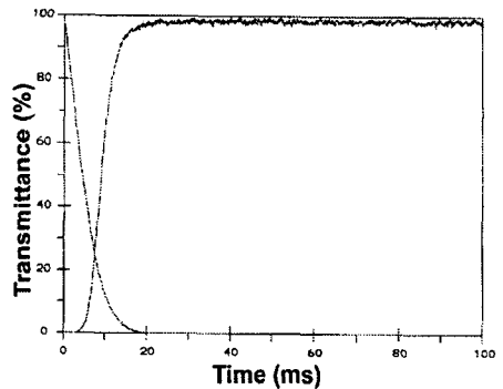
그림 5. 음의 보상 필름을 사용하지 않은 advanced VA-π 셀의 응답 특성.
