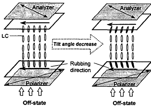
그림 3. Advanced VA-π 셀의 원리.
