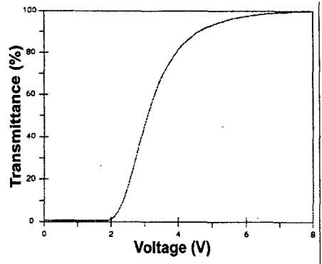
그림 4. 음의 보상 필름을 사용하지 않은 advanced VA-π 셀의 V-T 특성.
