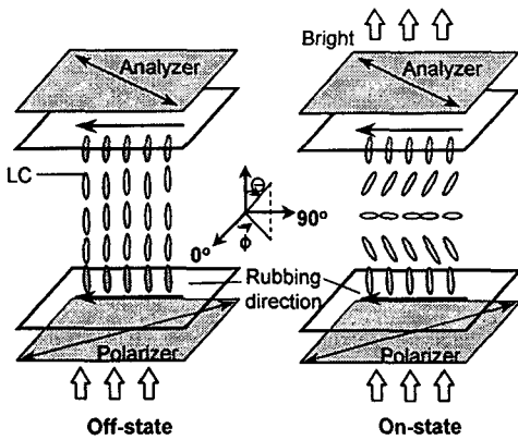
그림 2. 보상 필름을 사용하지 않은 VA-π 셀의 구조.
