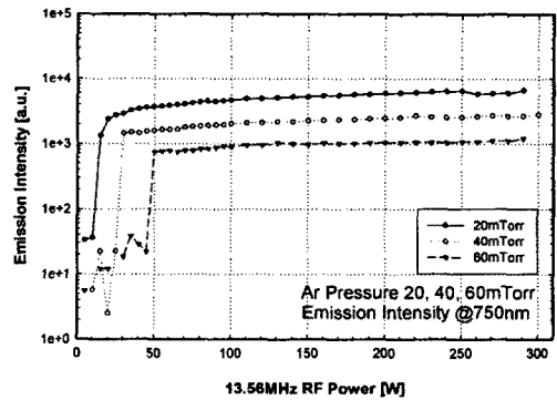
그림 5. Ar Gas 압력과 RF 전력 변화에 따른 Ar- I 라인인 750nm의 emission intensity Fig 5. Emission intensity (Ar- I 750) as a function of RF power variation for each gas pressure
