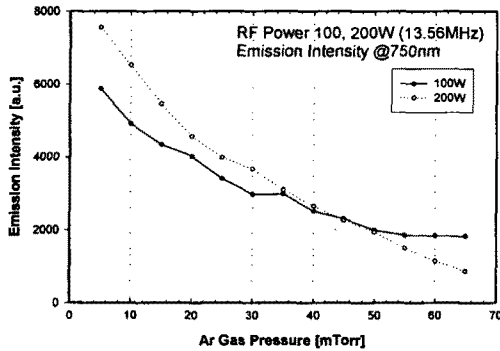
그림 3. Ar Gas의 750nm에서 emission intensity Fig 3. Emission intensity of Ar Gas at 750nm
