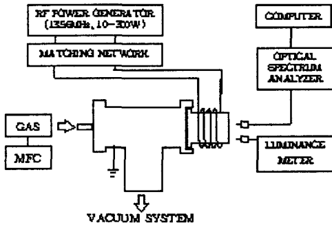
그림 1. 실험장치 개략도
