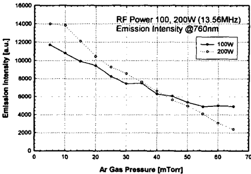
그림 4. Ar Gas의 760nm에서 emission intensity Fig 4. Emission intensity of Ar Gas at 760nm
