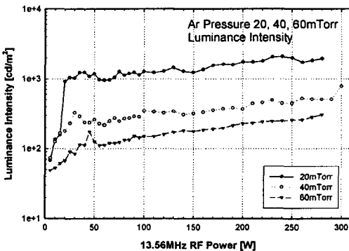
그림 7. Ar Gas 압력에서 RF 전력 변화에 따른 Ar-I 라인인 750nm의 휘도 측정 Fig 7. Luminance (Ar-I 750) as a function of power variation
