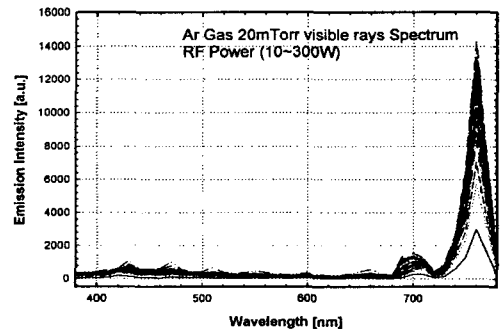
그림 2. Ar Gas의 Spectrum
