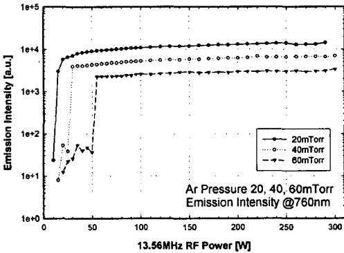
그림 6. Ar Gas 압력에서 RF 전력 변화에 따른 Ar-I 라인인 760nm의 emission intensity Fig 6. Emission intensity (Ar-I 760) as a function of RF power variation for each gas pressure
