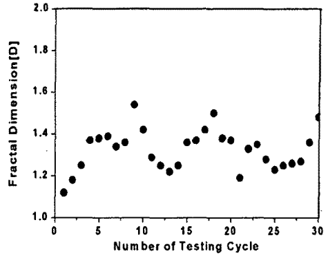
그림 4. EPDM 애자의 가속실험 결과(저비중)
