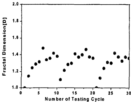
그림 3. 실리콘 애자의 가속실험 결과
