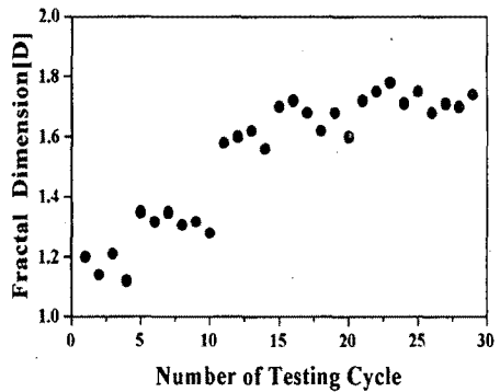
그림 6. EPDM 애자의 가속실험 결과(고비중)
