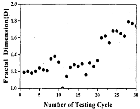
그림 5. EPDM 애자의 가속실험 결과 (고비중)
