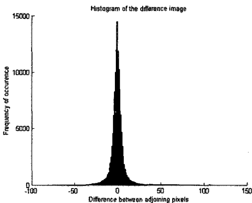
(b) 차분 영상의 히스토그램
