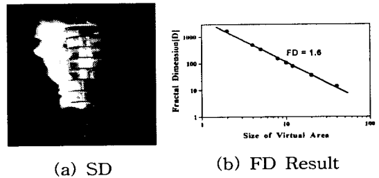
그림 1. 가속사이클 후에 발전된 SD 및 프랙탈 차원
