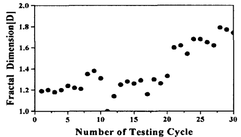
그림 5. EPDM 애자의 가속실험 결과 (고비중).
