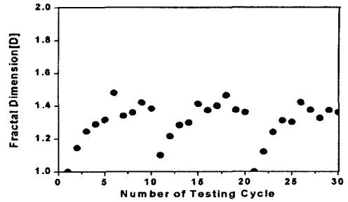
그림 3. 실리콘 애자의 가속실험 결과.
