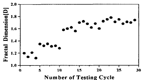
그림 6. EPDM 애자의 가속실험 결과 (고비중).
