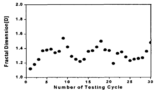
그림 4. EPDM 애자의 가속실험 결과 (저비중).
