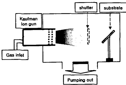
그림 1. IB 조사 시스템.
