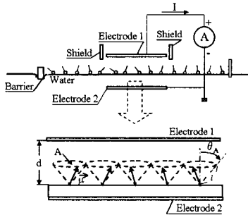
그림 1. 변위전류 측정장치
