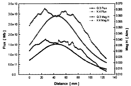
그림 3. 두께 변화에 따른 자속과 자계강도
