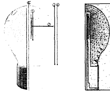
그림 1. 무전극 램프 형상과 내부도 및 요소분할.
