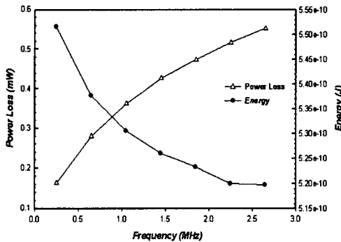
그림 4. 주파수변화에 대한 전력손실과 에너지 (Q-type)
