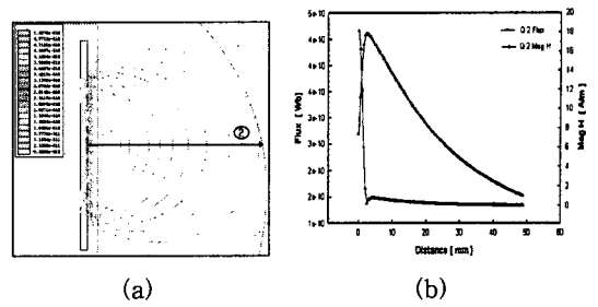
그림 2. (a) 자속 분포 & (b) 선 2에서의 자속과 자계 강도 (Q type)
