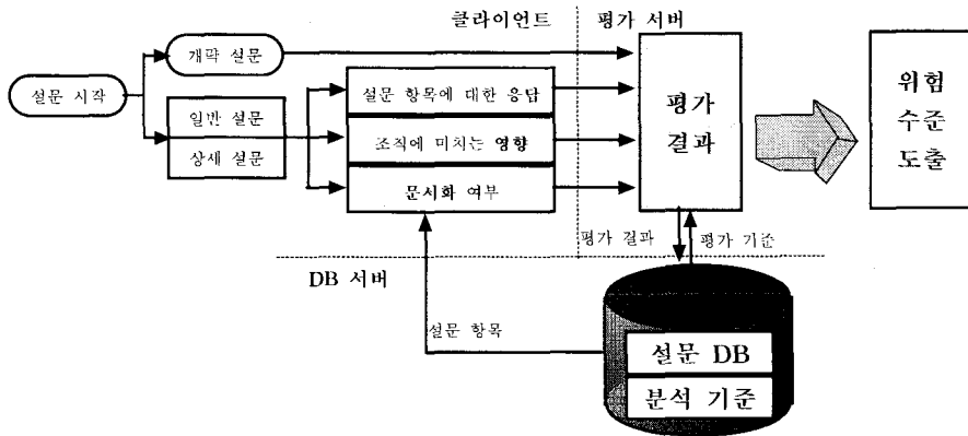
<그림 1> 설문 처리과정
