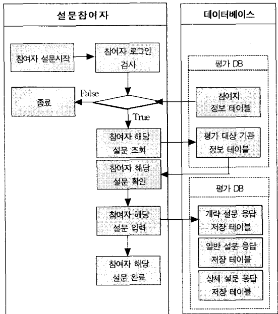
<그림 3> 절차의 DB테이블의 관계
