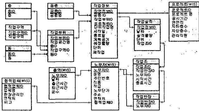
그림 10 데이터 베이스 모델
