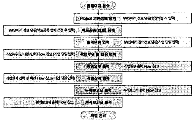
그림 8 S-SMART 시스템 MASTER FLOW
