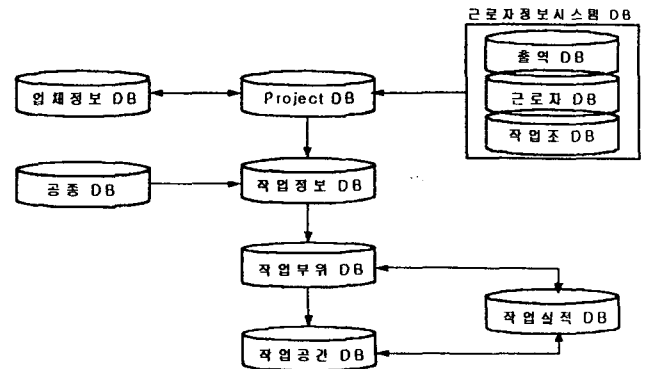
그림 9 데이터 베이스 구성도
