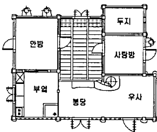
그림 7. 권영해씨 집 평면
