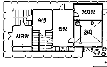
그림 8. 채충기씨 집 평면
