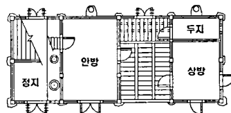
그림 6. 종택 평면
