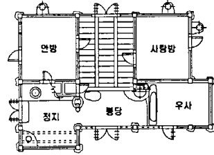
그림 4. 전형적인 여칸집 평면(황후규씨 집)
