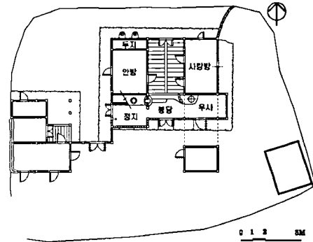
그림 1. 임차노미씨 집 배치·평면도
