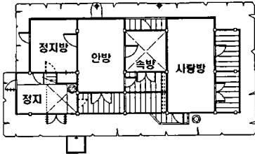
그림 10. 채희술씨 집 평면
