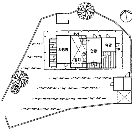
그림 3. 채희진씨 집 배치·평면도
