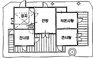
그림 11. 채상식씨 집 평면
