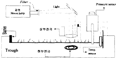
그림 3. 수면위의 광자적 전달에 따른 변위전류 측정장치 Fig. 3. Displacement current measuring apparatus according to light stimulus transfer on water surface
