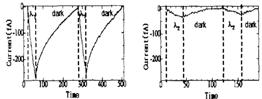
그림 6. AZ-G4의 광조사( \lambda_1=365\text{nm}, \lambda_2=450\text{nm} ) Fig. 6. Photomodulation of AZ-G4( \lambda_1=365\text{nm}, \lambda_2=450\text{nm} )
