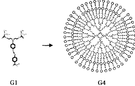
그림 2. AZ-G4의 분자 구조 Fig. 2. Molecule structure of AZ-G4
