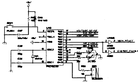
그림 6 UPS/상용 디스플레이부
