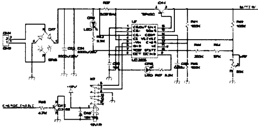
그림 2 배터리 충전부
