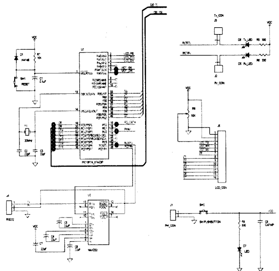
그림 1 무정전 전원장치의 마이컴 제어부
