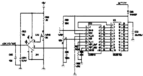
그림 3 배터리 잔여량 디스플레이부
