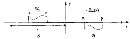
그림 5 슬롯영역에서의 임의 자속밀도분포
