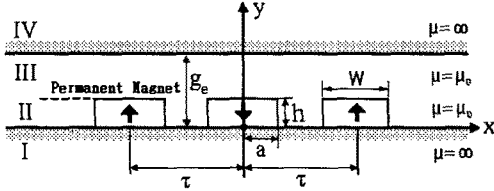
그림 2 영구자석에 의한 자계 해석모델
