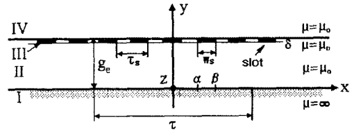
그림 4 슬롯의 가상등가자화전류 모델
