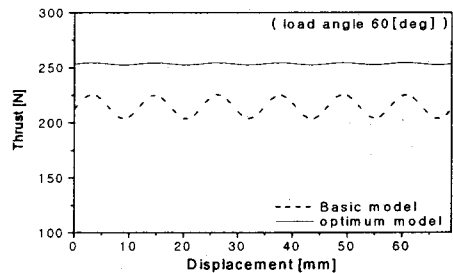
그림 9 정상상태 운전 특성
