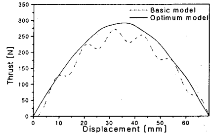
그림 8 추력특성
