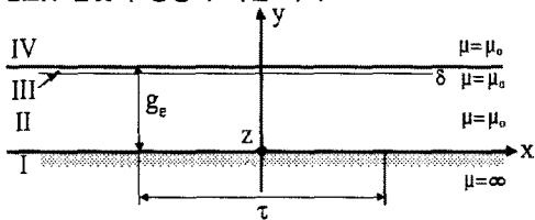
그림 3 평활철심 표면의 등가자화전류 모델
