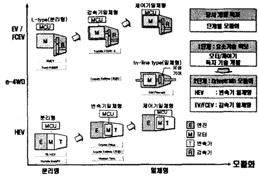
그림 7 환경차량용 전기식 Powertrain
