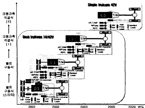
그림 6 42V시스템의 기술단계
