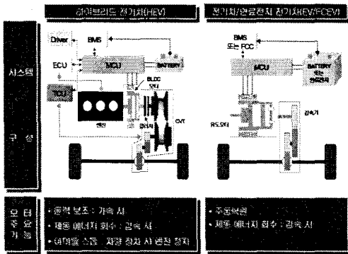
그림 5 환경차량의 시스템 구성 및 기능
