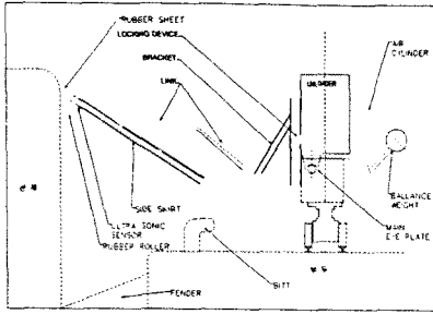
그림 1. System Layout
