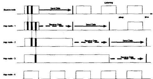
그림 1. 변형된 listen / sleep 기법 Fig. 1. Modified listen / sleep duty cycle
