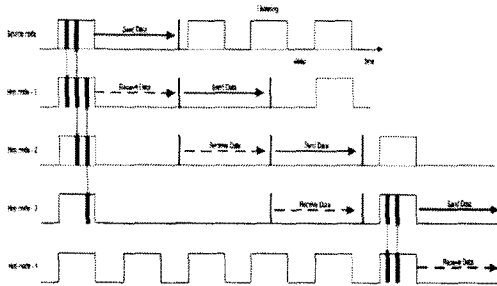
그림 2. 과도 listen 상태를 제거
