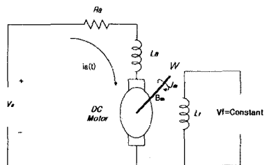
그림 1. 직류서보전동기의 등가회로.
