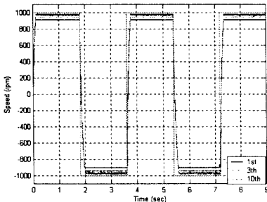
그림 7. 부하외란이 존재할 때 직류서보전동기의 속도 응답. Fig. 7. DC servo motor drive speed response due to the load disturbance.
