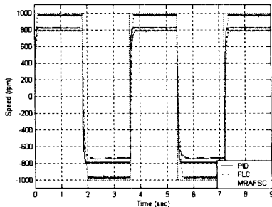
그림 7. 부하외란이 존재할 때 직류서보전동기의 속도 응답. Fig. 7. DC servo motor drive speed response due to the load disturbance.
