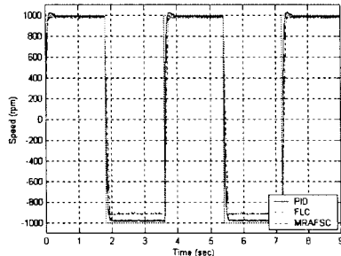
그림 6. 부하외란이 존재하지 않을 때 PID, FLC 와 MRAFSC 직류서보전동기의 속도 응답. Fig. 6. PID, FLC and MRAFSC DC servo motor drive speed response (no load).
