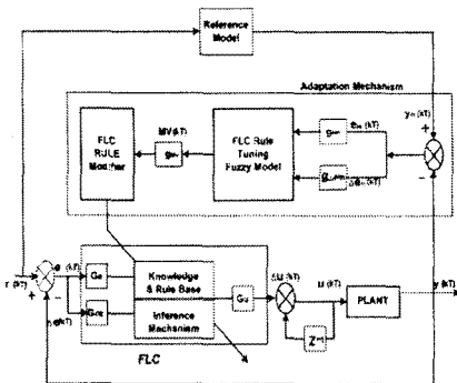
그림 3. MRAFSC의 블록선도
