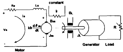
그림 5. 직류서보 제어 시스템의 구성도
