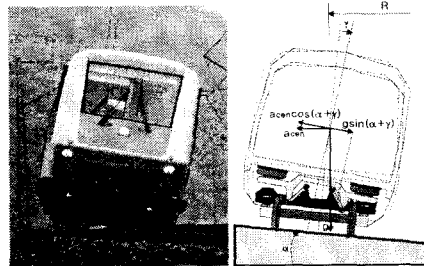
그림 1 틸팅차량의 횡가속도 저감의 원리
