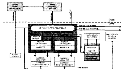
그림 4 차량시스템 인터페이스
