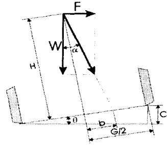
그림 2 곡선부 원심력과 중력의 합력관계
