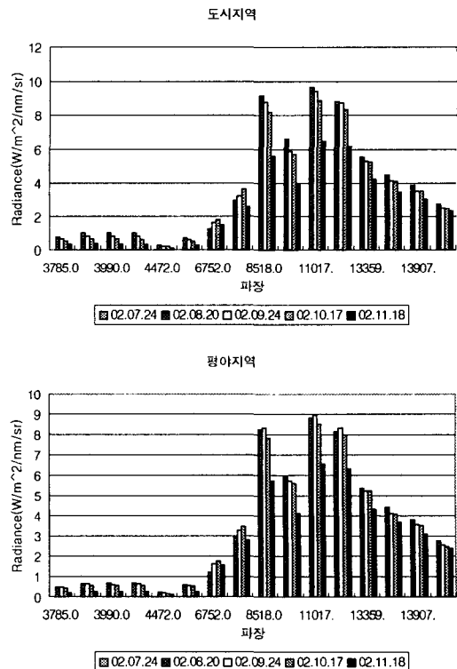
그림3.4(a) Thermal Emission Bands에서 도시지역, 평야지역에 대한 월별 파장별 TOA radiance 분포.
