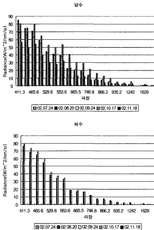
그림3.3(b) Reflectance Solar Bands에서 담수, 해수에 대한 월별 파장별 TOA radiance 분포
