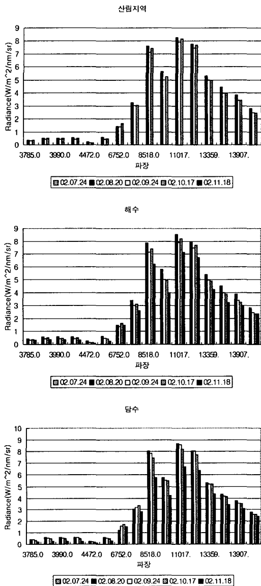
그림3.4(b) Thermal Emission Bands에서 산림지역, 해수, 담수에 대한 월별 파장별 TOA radiance 분포.
