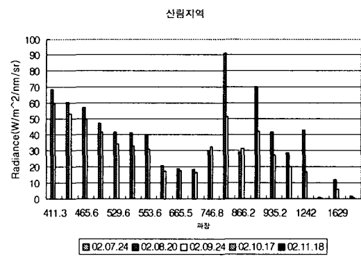
그림3.3(a) Reflectance Solar Bands에서 도시지역, 평야지역, 산림지역에 대한 월별 파장별 TOA radiance분포
