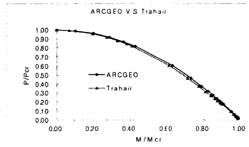
그림 4 ARC GEO와 이론식의 비교
