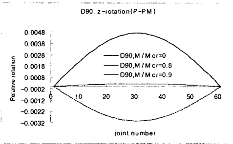
그림 17 Z-축 상대모드(D90,P-PM)
