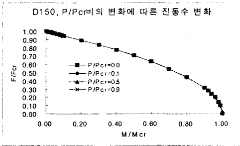
그림 11 축력비에 따른 진동수 변화(D150,P-PM)
