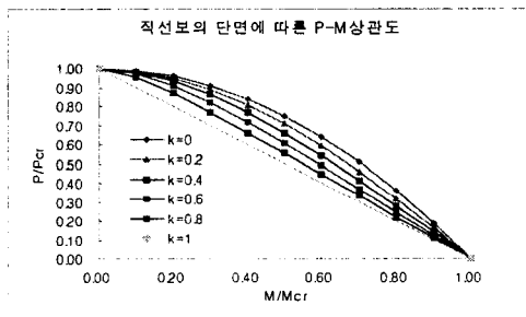
그림 3 단면변화에 따른 P-M상관도
