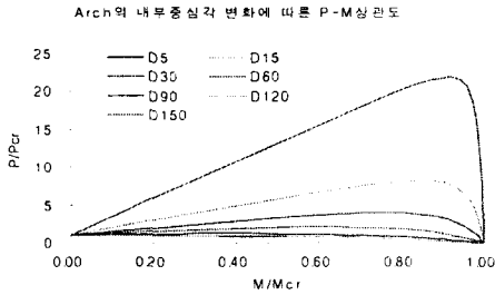
그림 8 내부중심각의 변화에 따른 P-M상관도(등분포압축및정모멘트)
