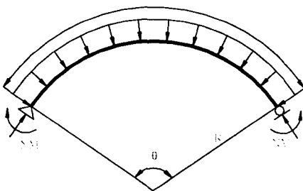
그림 1 등분포 압축 및 부모멘트
