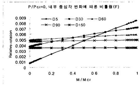
그림 14 내부 중심각에 따른 최대비틀림(P-NM)
