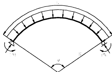
그림 2 등분포 압축 및 정모멘트
