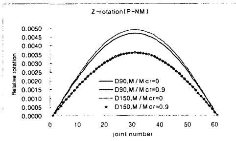
그림 13 Z-축 상대변위(P-NM)
