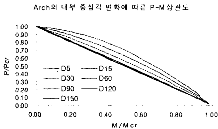
그림5 내부중심각의 변화에 따른 P-M상관도(등분포 압축및부모멘트)
