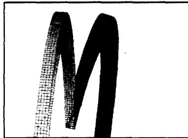
그림6 곡률면의 좌굴형상(등분포 압축및부모멘트)
