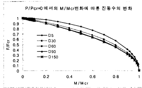
그림 12 모멘트비에 따른 진동수 변화(P-PM)
