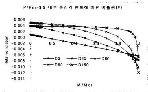
그림 18 내부중심각에 따른 최대 비틀림(P-PM)
