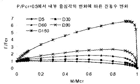
그림 16 내부 중심각에 따른 진동수 변화(P-PM)
