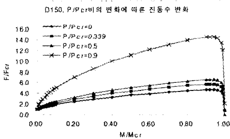
그림 15 축력비에 따른 진동수 변화(D150,P-PM)
