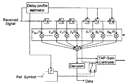
그림 2. 적응형 등화기
