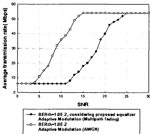
그림7. 적응변조 OFDM 시스템에서 전송효율
