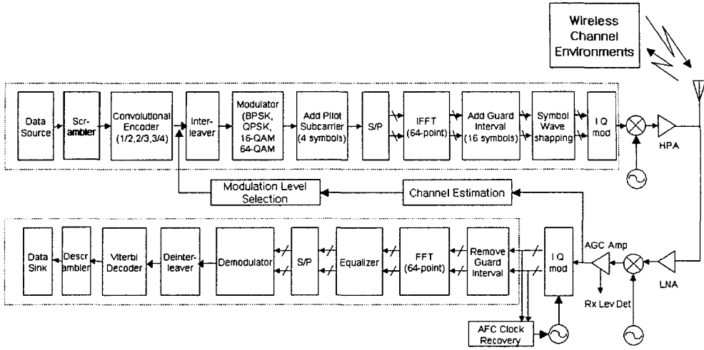
그림 1. 적응형 등화기를 적용한 적응변조 OFDM 시스템
