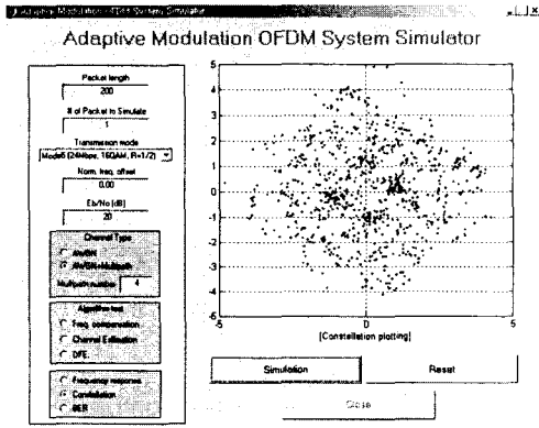
그림 3. OFDM/16QAM 시스템에서의 성좌점 시뮬레이션 (Multipath fading, Eb/No=20dB)
