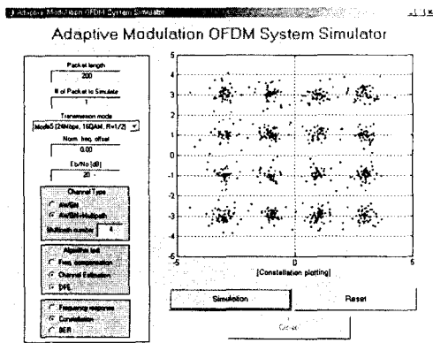
그림 4. OFDM/16QAM 시스템에서 등화기 적용 후의 성좌점 시뮬레이션 (Multipath fading, Eb/No=20dB)
