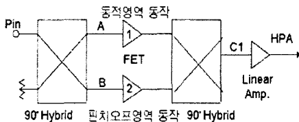
그림 2. 공통 게이트 방식의 MESFET 전치 왜곡기 Fig. 2 .MESFET predistortor using commom gate circuit.
