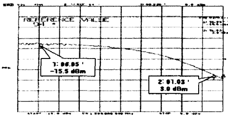
그림 7. (b) 전치왜곡기를 사용한후의 위상의 변화 Fig 7. (b) Phase variation with predistortion
