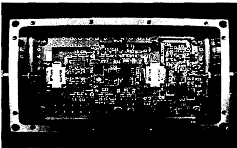
그림 5. 제작된 전치왜곡기 Fig. 5. The constructed predistorter.
