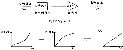
그림 1. 전치 왜곡 방식의 동작 원리 Fig. 1. Principle of predistortion.
