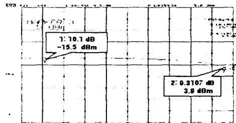
그림 7.(a) 전치왜곡기를 사용한후의 진폭의 변화 Fig 7.(a) Amplitude variation with Predistorter
