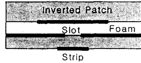
(b) SSFIP 구조
