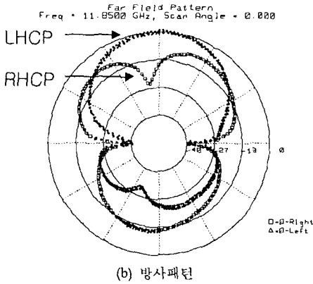
그림 2. 1x3 기본 안테나의 반사계수와 방사패턴 (시뮬레이션 결과)
