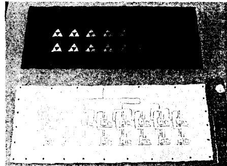
그림 5. 제작된 8x2 배열 안테나
