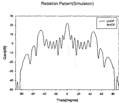
그림 4. 8x2 배열 안테나의 방사패턴 (시뮬레이션 결과)
