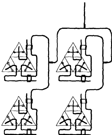
그림 3. 2x2 배열 안테나
