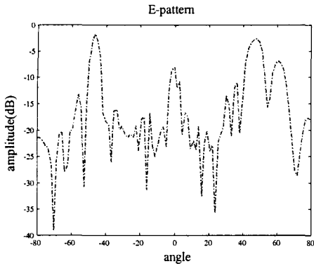
그림 7. 8x2 배열 안테나의 방사패턴 측정 결과
