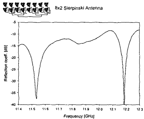
그림 6. 8x2 배열 안테나의 반사계수 측정 결과
