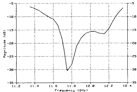
(a) 반사계수
